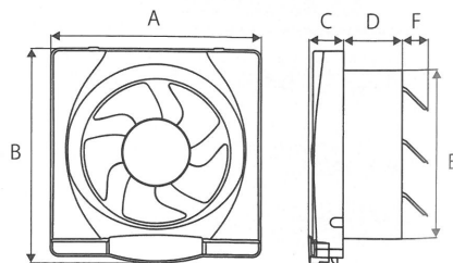
寸法図
