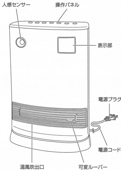
前面
