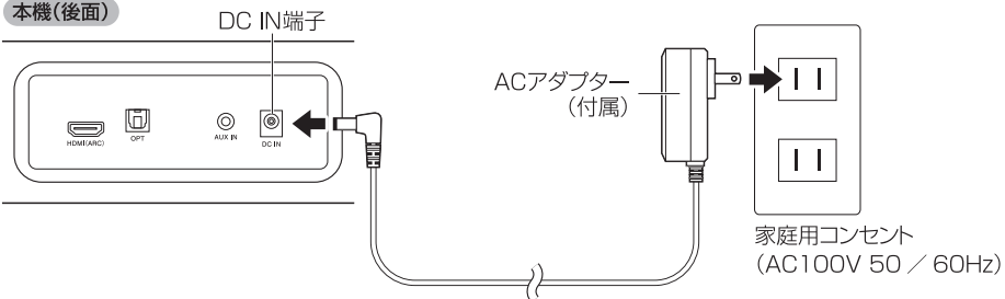
本機(後面)
