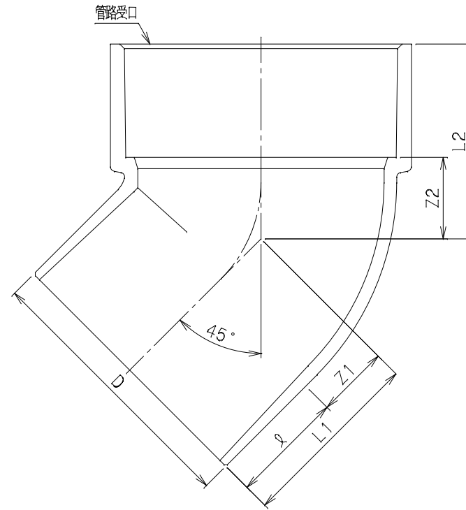
呼び径 50
