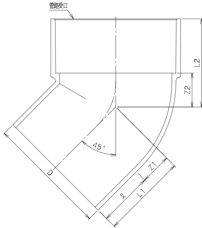
呼び径 40, 75, 100
