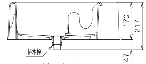
排水栓組立完成図
