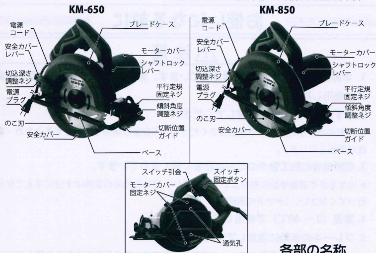
各部の名称
