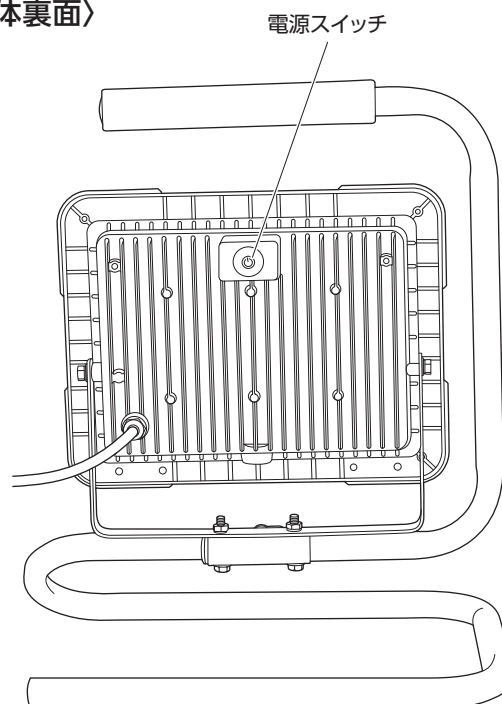
〈本体裏面〉
