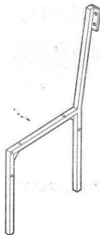
③ チェア左フレーム × 1
