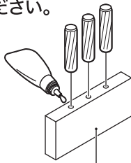
⑩ 支え板×2
