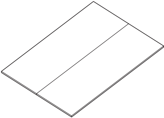
⑤ 背板 × 1
