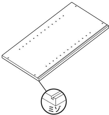
① 側板 ×2
