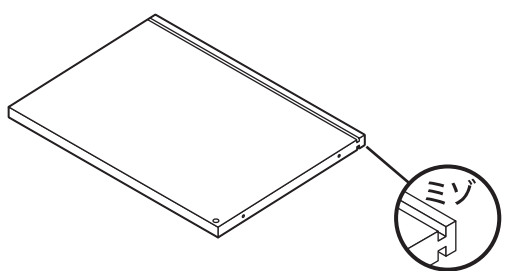
⑦ 固定棚 × 3
