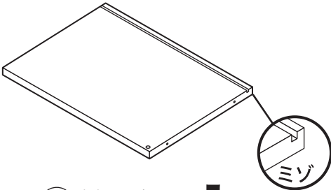
④ 地 板 × 1
