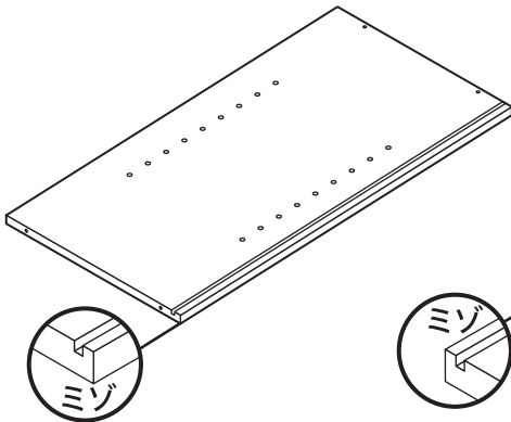
⑥ 上左側板 × 1
