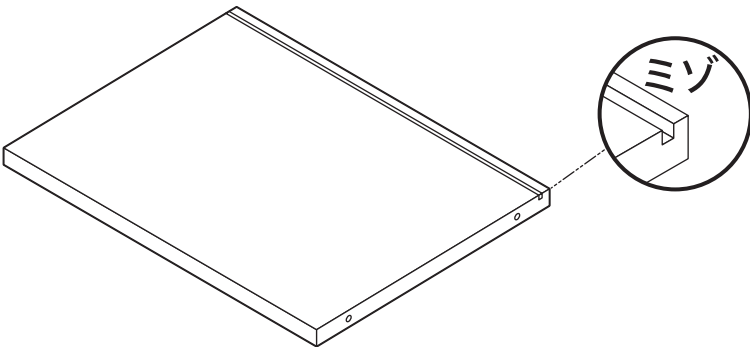
③ 天地板 × 2
