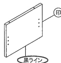
④ 左側板
