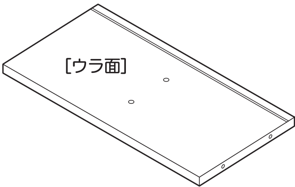
① 天地板 ×2
